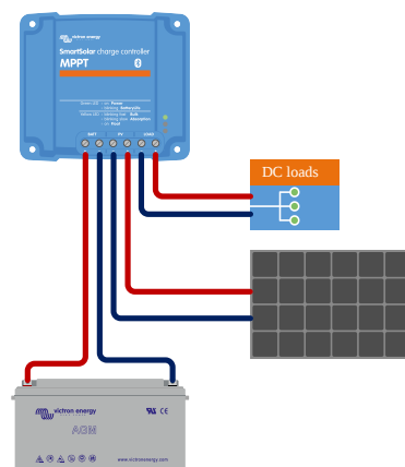
Sistema de cargador solar con cargas CC conectadas a la salida de carga
