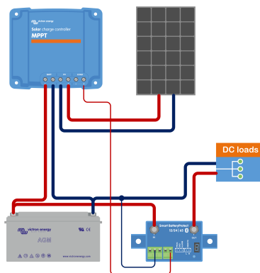
Sistema de cargador solar con cargas CC conectadas directamente a la batería mediante un BatteryProtect controlado por la salida de carga
