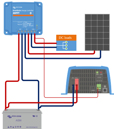
Sistema de cargador solar con inversor conectado directamente a la batería y controlado por la salida de carga
